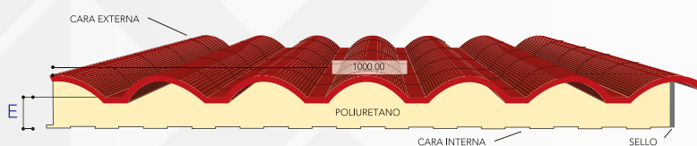
METCOPPO
